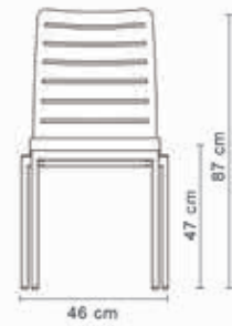
08/1 Tiefe 55,5 cm Gewicht 6,2 kg Stuhlstapel 10
